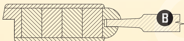
profil, rám č. 2
