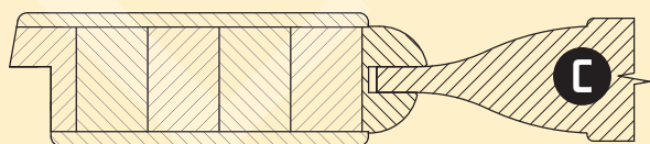
profil, rám č. 2
