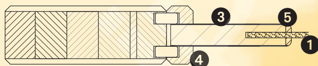
osadenie výplne a skla, Aneta
