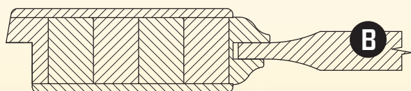
profil, rám č. 1
