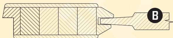
profil, rám č. 3
